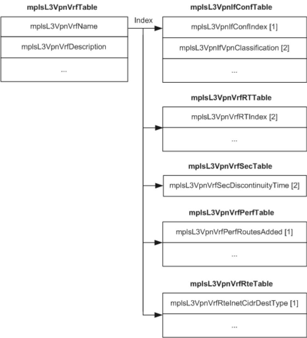
图 158-1 L3VPN MIB 中的表间关系图
